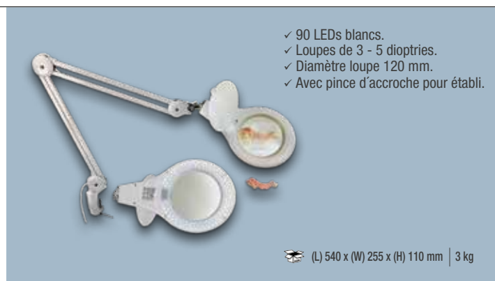
Loupe avec éclairage LED
