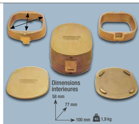
Moule carré
