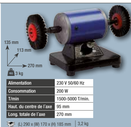
Mini tour à polir vitesse variable Réf. 100277
