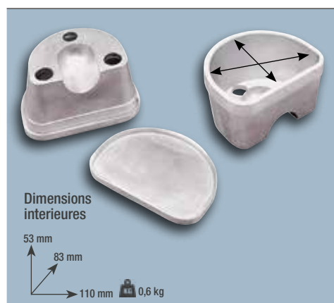
Cuvette (grand modèle) Réf. 020150 Matériau: Aluminium
