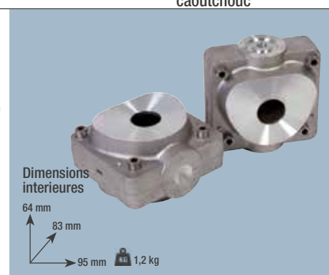
Cuvette (à gel pour injecter polyamides) Réf. 020210 Matériau: Aluminium
