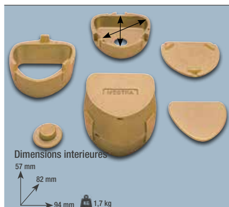
Moule triangulaire
