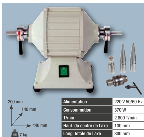
Tour à polir Import Réf. 100274
