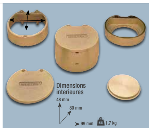
Moule rond
