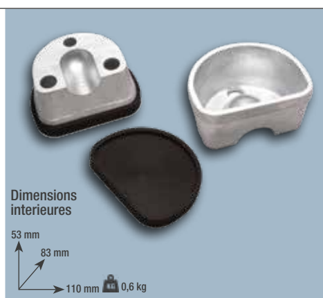
Cuvette (grand modèle) Réf. 020151 Matériau: Aluminium - Caoutchouc
