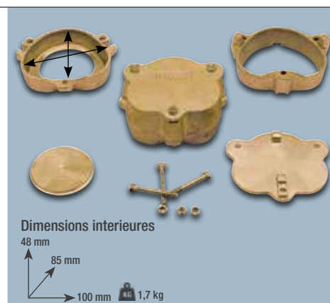
Moule à vis (avec éjecteur)
