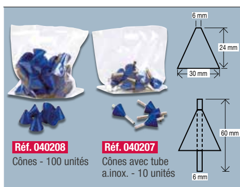
Cônes de polyéthylène
