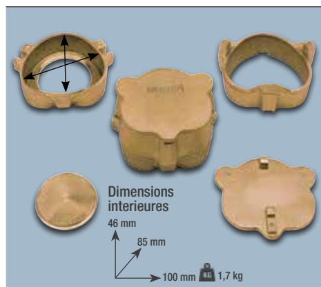
Moule sans vis (avec éjecteur)
