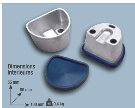
Cuvette (petit modèle) Réf. 020171 Matériau: Aluminium - Caoutchouc
