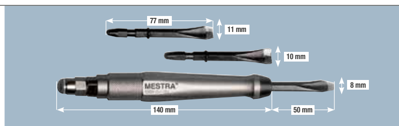
Burin pneumatique Réf. 050550
