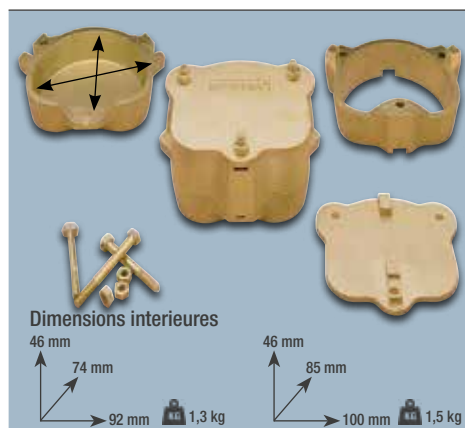
Moule à vis
