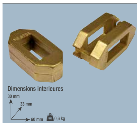
Moule pour bridges
