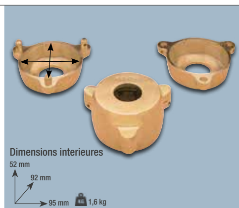
Moule à trois becs (pour bride)
