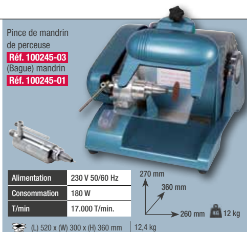
Tour à polir à grande vitesse Réf. 100245
