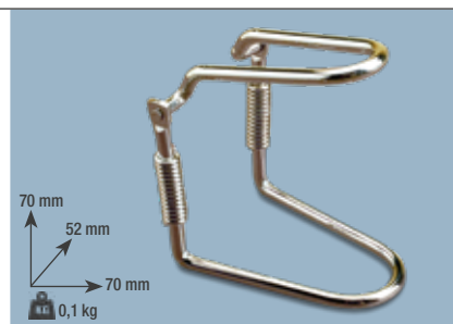
Articulateur à ressorts
