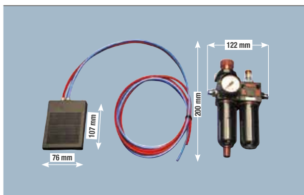
Pédale pour burin pneumatique Réf. 050552
